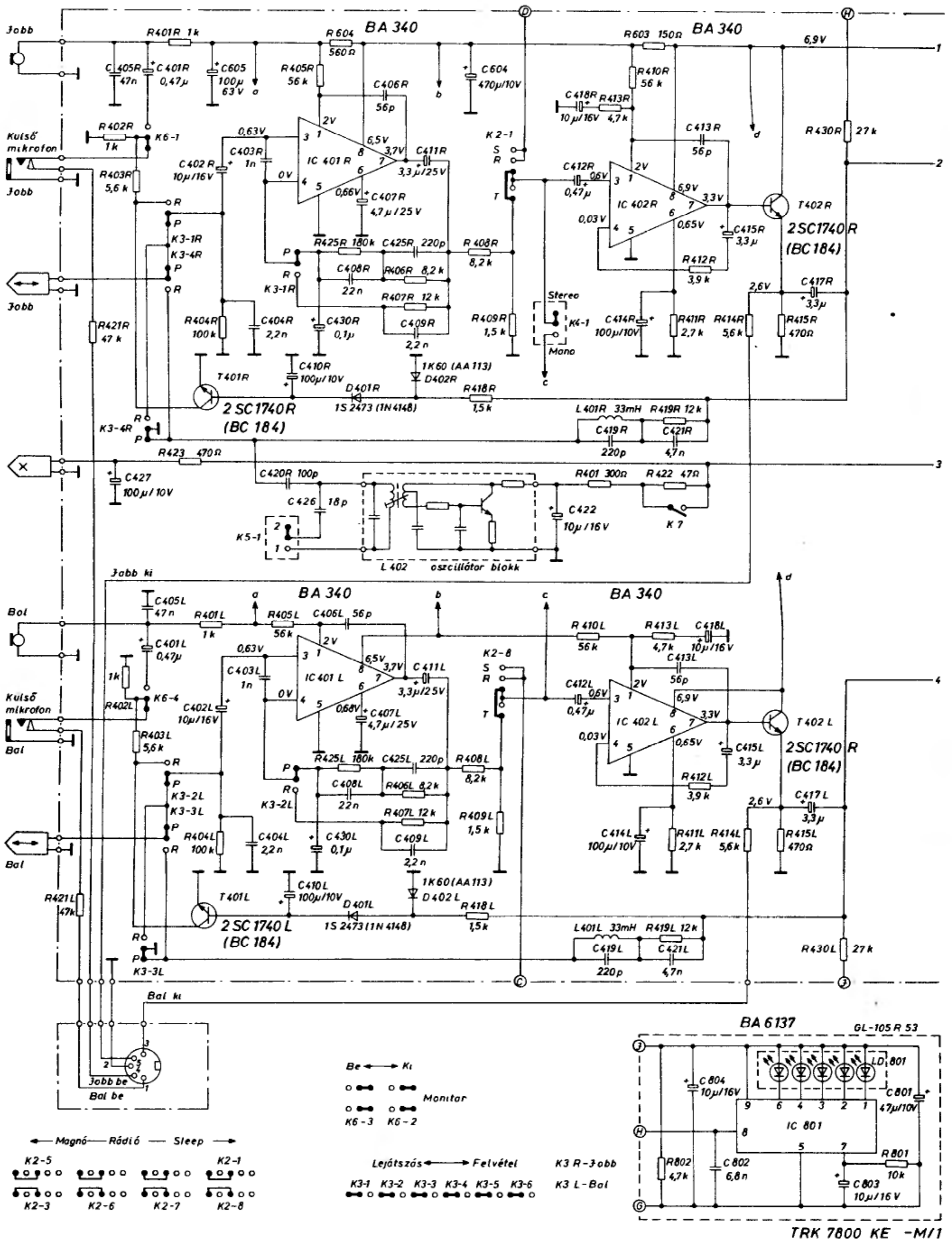
143. ábra A Hitachi TRK—7800 KE áramköreinek kapcsolási vázlatja
